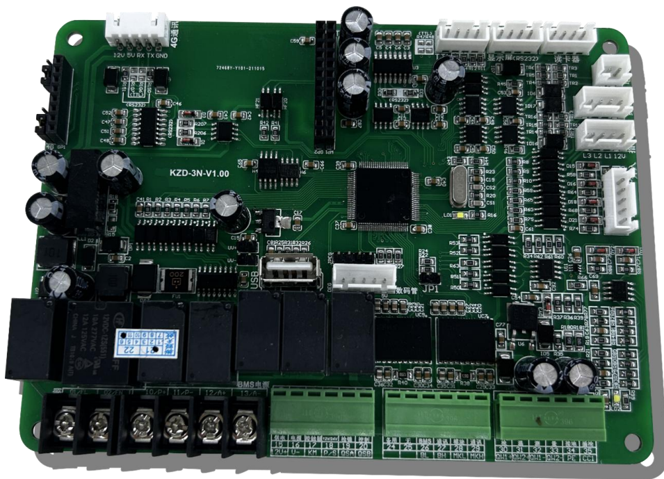
ZGKZD-3N 直流单充控制器 接线端子图
