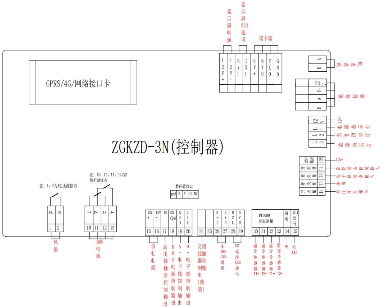
ZGKZD-3N 直流单充控制器 接线端子图
